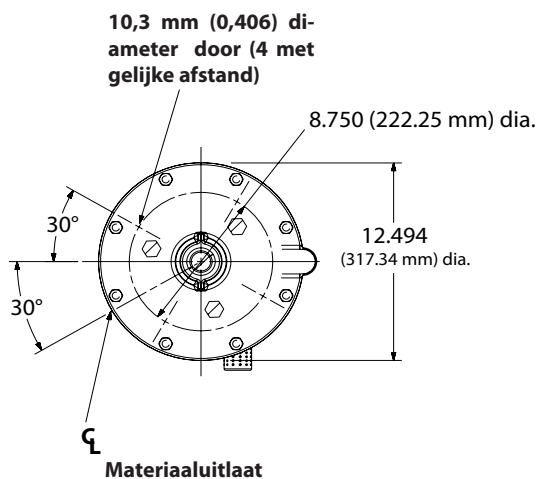
ONDERAANZICHT
