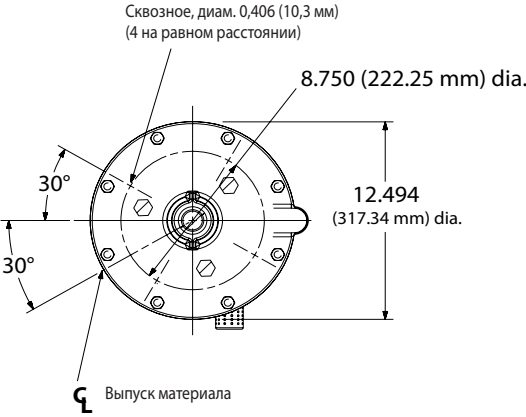
ВИД СНИЗУ
