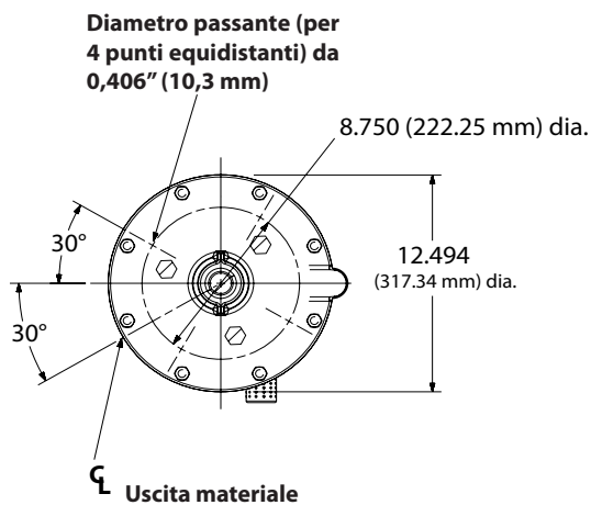
VISTA INFERIORE
