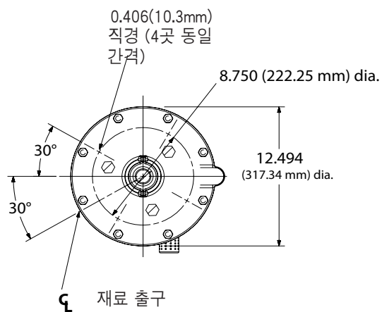
하단 보기
