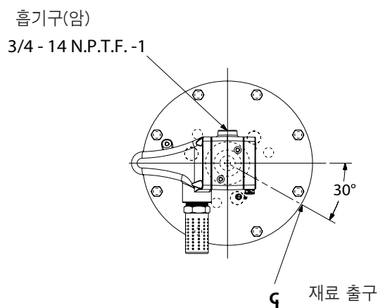
상위 뷰
