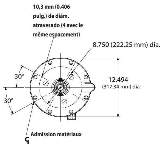
VUE INFÉRIEURE
