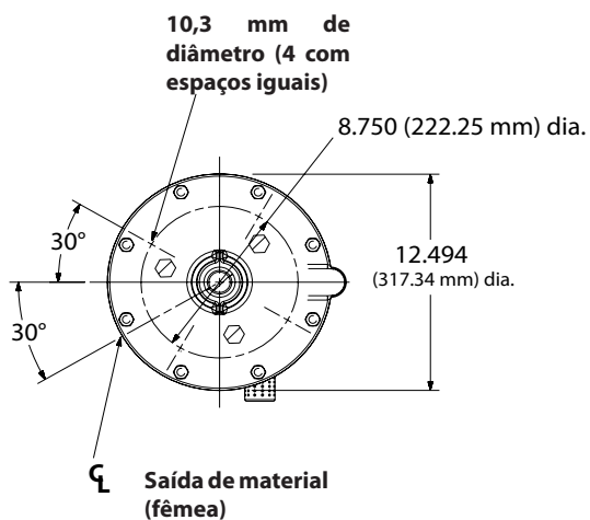
VISTA INFERIOR
