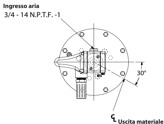
VISTA DALL'ALTO
