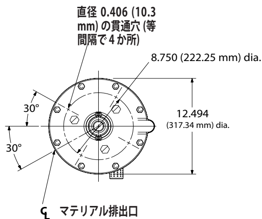
底面ビュー
